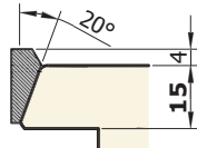
Terminale T 2545.20°
