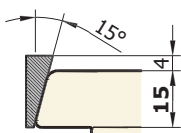
Terminale T 1255.15
