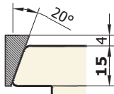
Terminale T 1255.20
